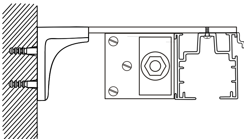
Стеновой монтаж
