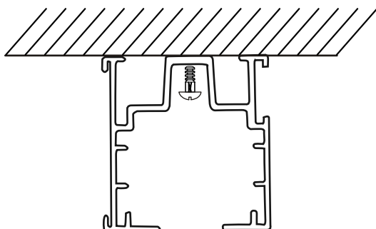
Потолочный монтаж
