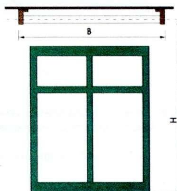
Монтаж к потолку над окном
