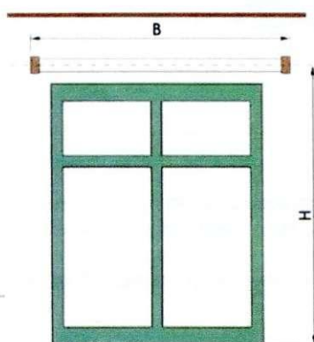
Монтаж к стене над окном
